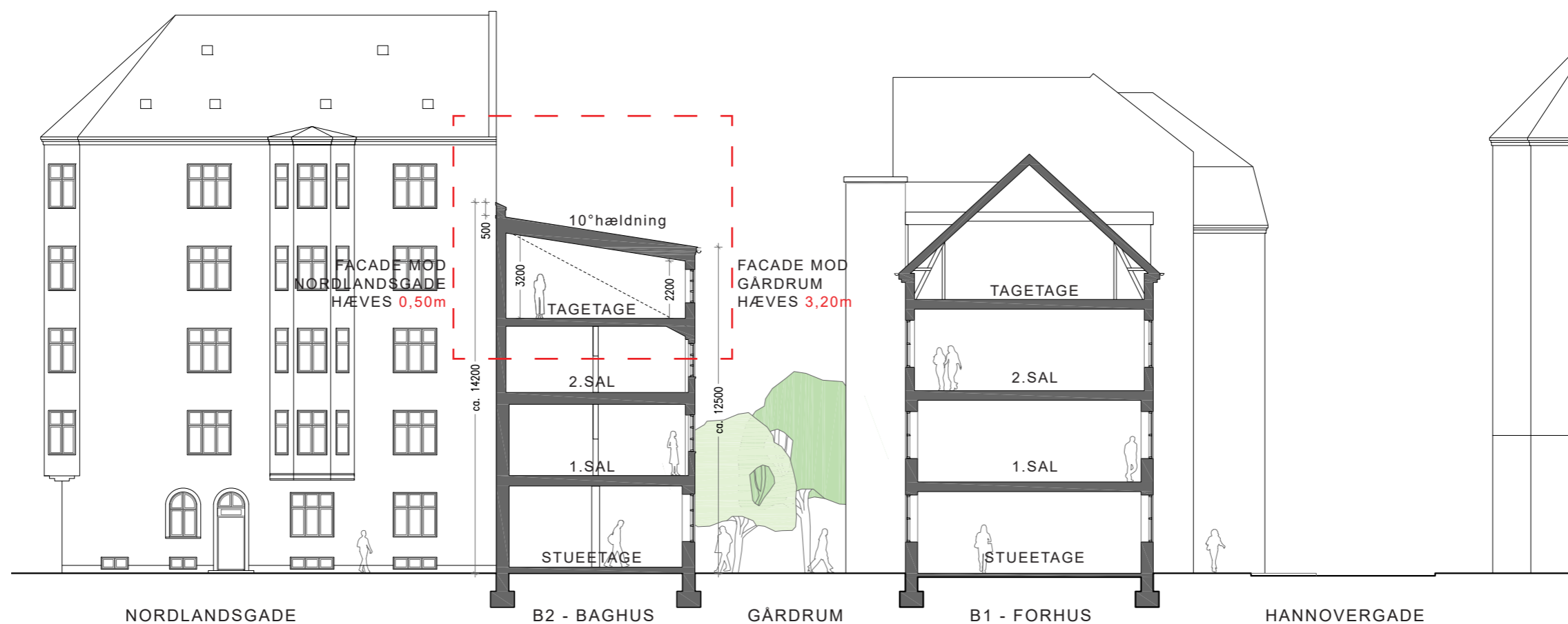
TVÆRSNIT - NORDLANDSGADE / HANNOVERGADE FORSLAG B
