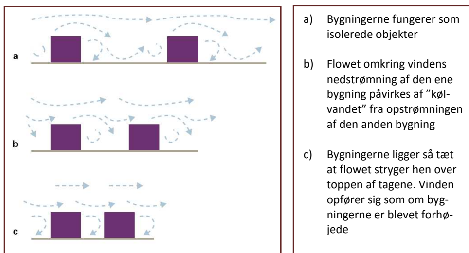
FIGUR 3: VINDENS FLOW OMKRING BYGNINGER. (CARBON TRUST 2008)
