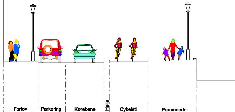
Tværprofil dobbeltrettet cykelsti
