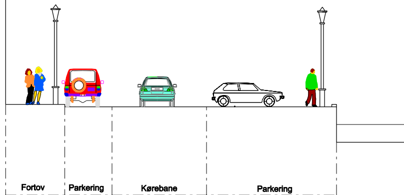
Eksisterende tværprofil Nyhavn
