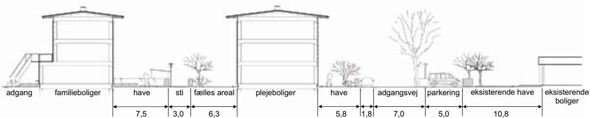
Snit B-B
