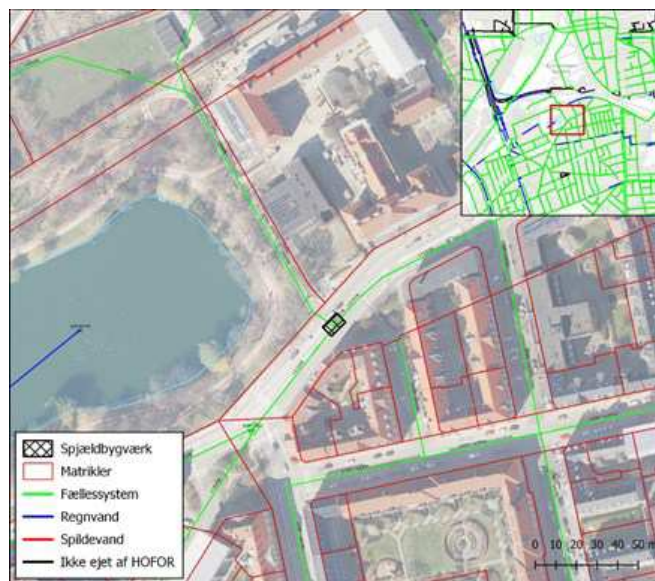
Figur 2: Nyt reguleringsbygværk i Bellmangsgade, som vandet kan opmagasineres og forsinkes bagved. Etablering af bygværket vil føre til at vandtilførslen mod Pumpestation Strandvænget kan reguleres – så frekvensen af overløb fra pumpestationen, inkl. overløb til Svanemøllebugten via UØ14.1, kan reduceres.
