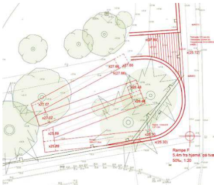
Figur 2 Rampe F, rampen begynder 5,4 m fra hjørnet, 50%, samlet rampe-længde 55m (og kræver fældning af to træer)
