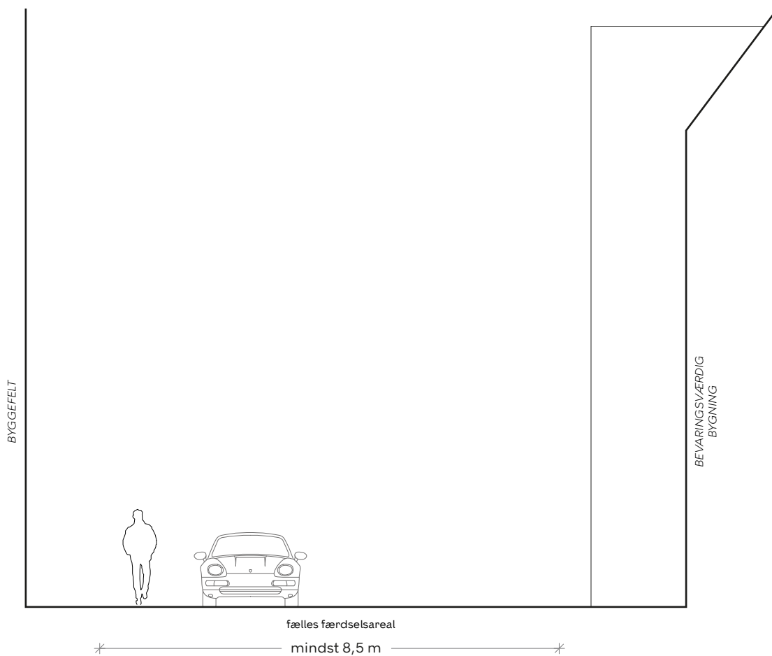
Snit A-A
