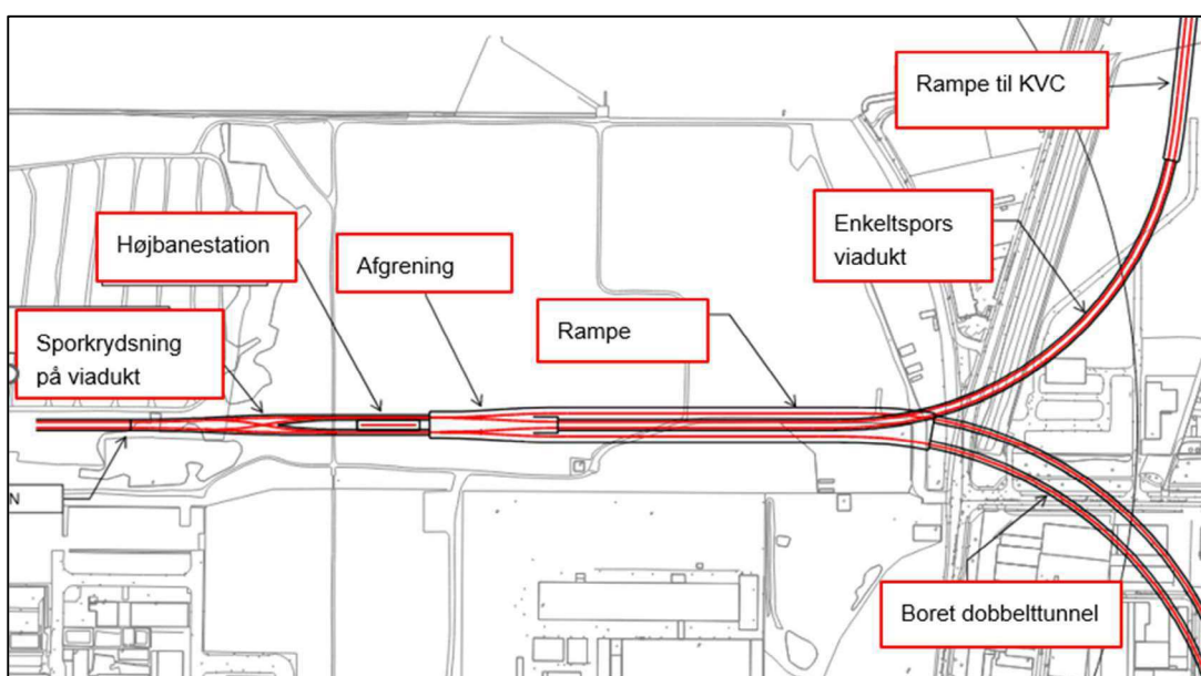
Figur 1: Placering af ramper, tunneler, viadukter og højbanestation v/Prags Boulevard. Placeringen er foreløbig og kan blive ændret.
