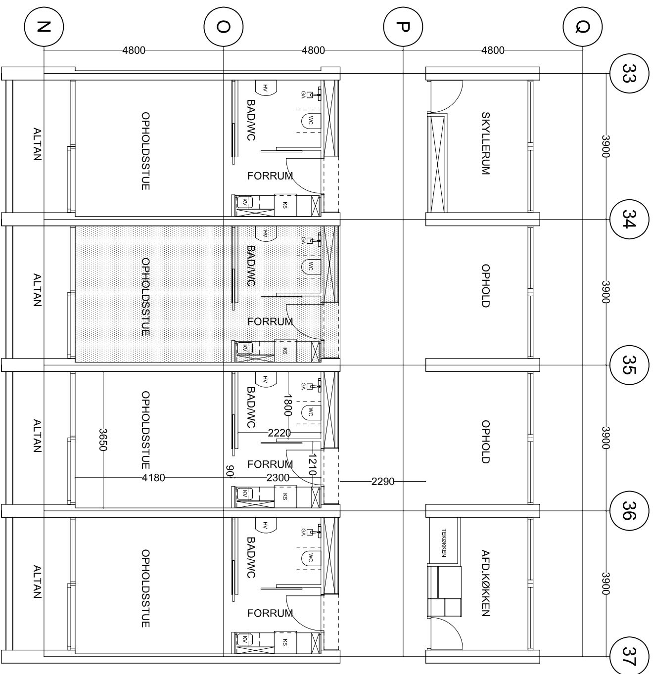
2. - 5. SALS PLANUDSNIT EKISTERENDE FORHOLD MÅL 1:100
