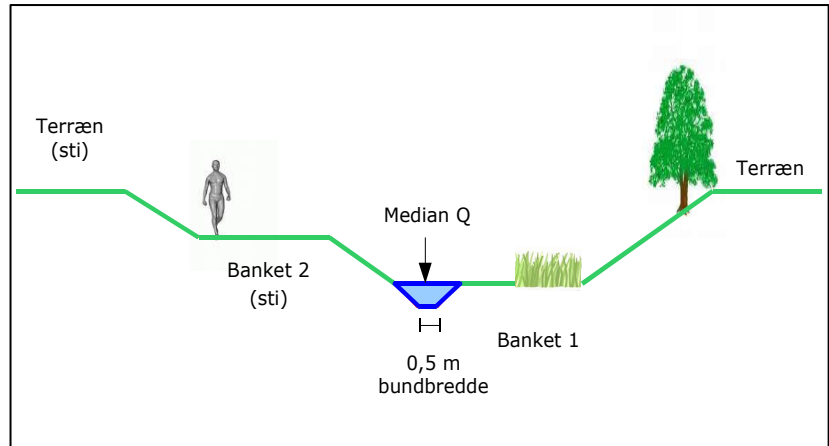
Figur 16: Princip for dobbeltprofil
