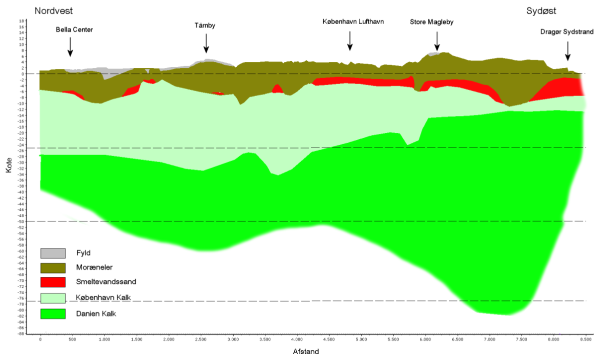
Figur 14.1 Geologisk profil 27
