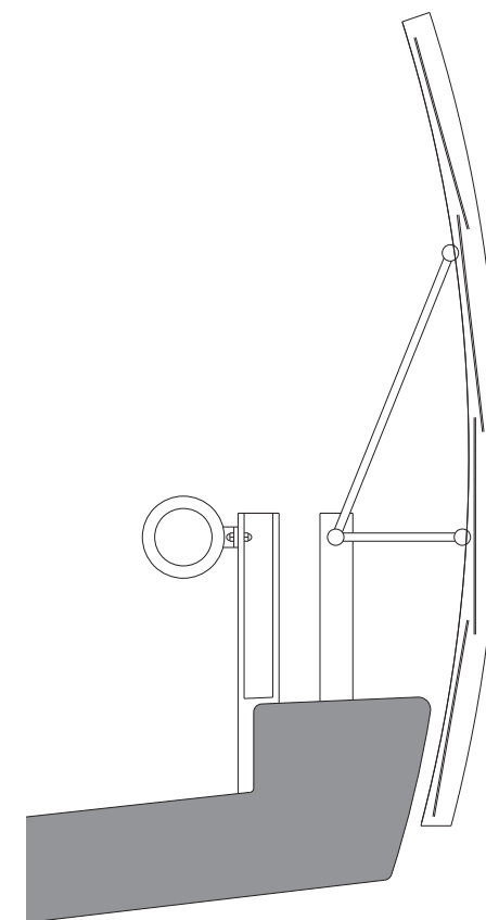
detalje støjskærm flyover 1:20
