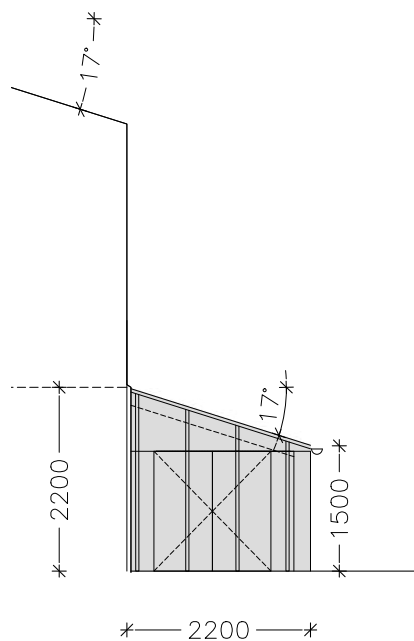
Skure udføres med samme tag- og facadedetaljering som på rækkehuse. Tag i samme hældning som rækkehuse. Skure udføres som trækonstruktion
