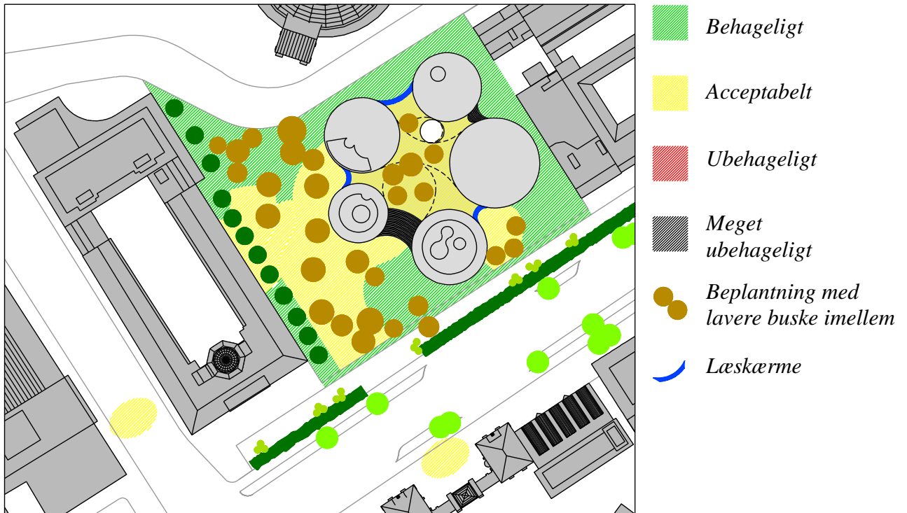
Figur 0.4. Illustration af vindmiljø i fokusområderne ved Axeltorv ved ny bebyggelse, med forbedret lokal lægivning.
