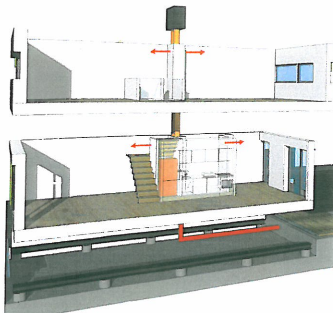
Basisbolig - installationsprincip. Illustration: ONV Arkitekter
