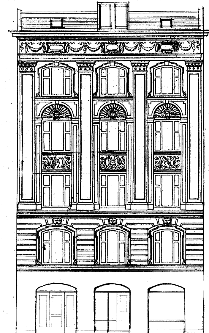
Facade.
