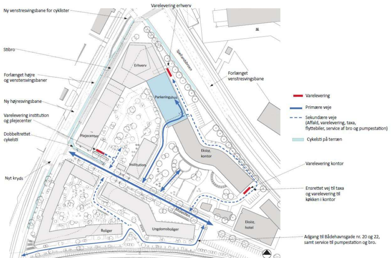
Figur 5-3 Situationsplan med det interne vejnet markeret (ikke opdateret i forhold til sti langs Bådehavngade /22).
