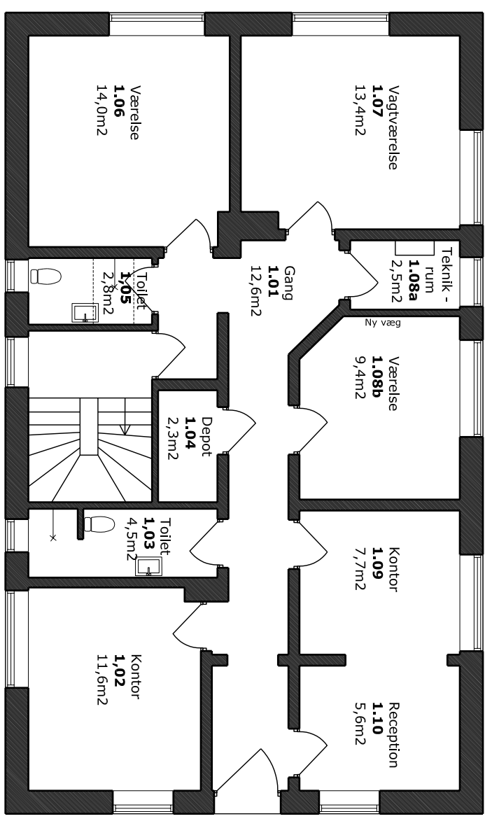
Fremtidig bygning B Stueplan
