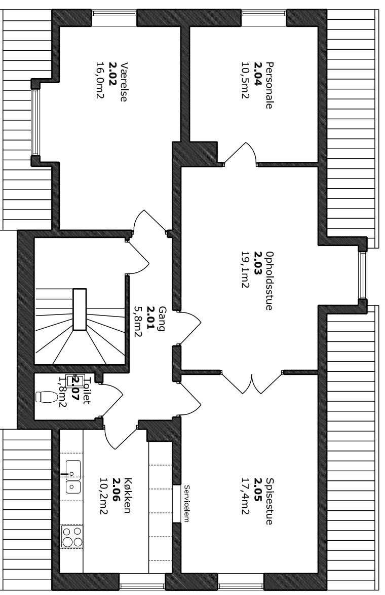
Fremtidig bygning B 1. sal
