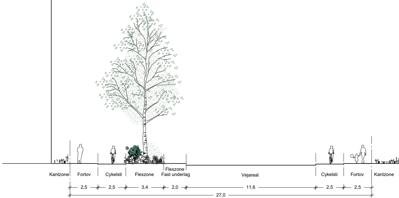
AA1 Vejtype a, snit AA1
