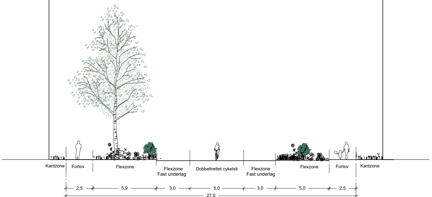
AA2 SCENARIO A Vejtype b, snit AA2
