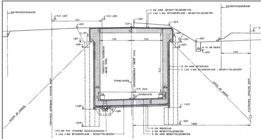
Figur 5.19 Tværsnit i Farumbanetunnelen
