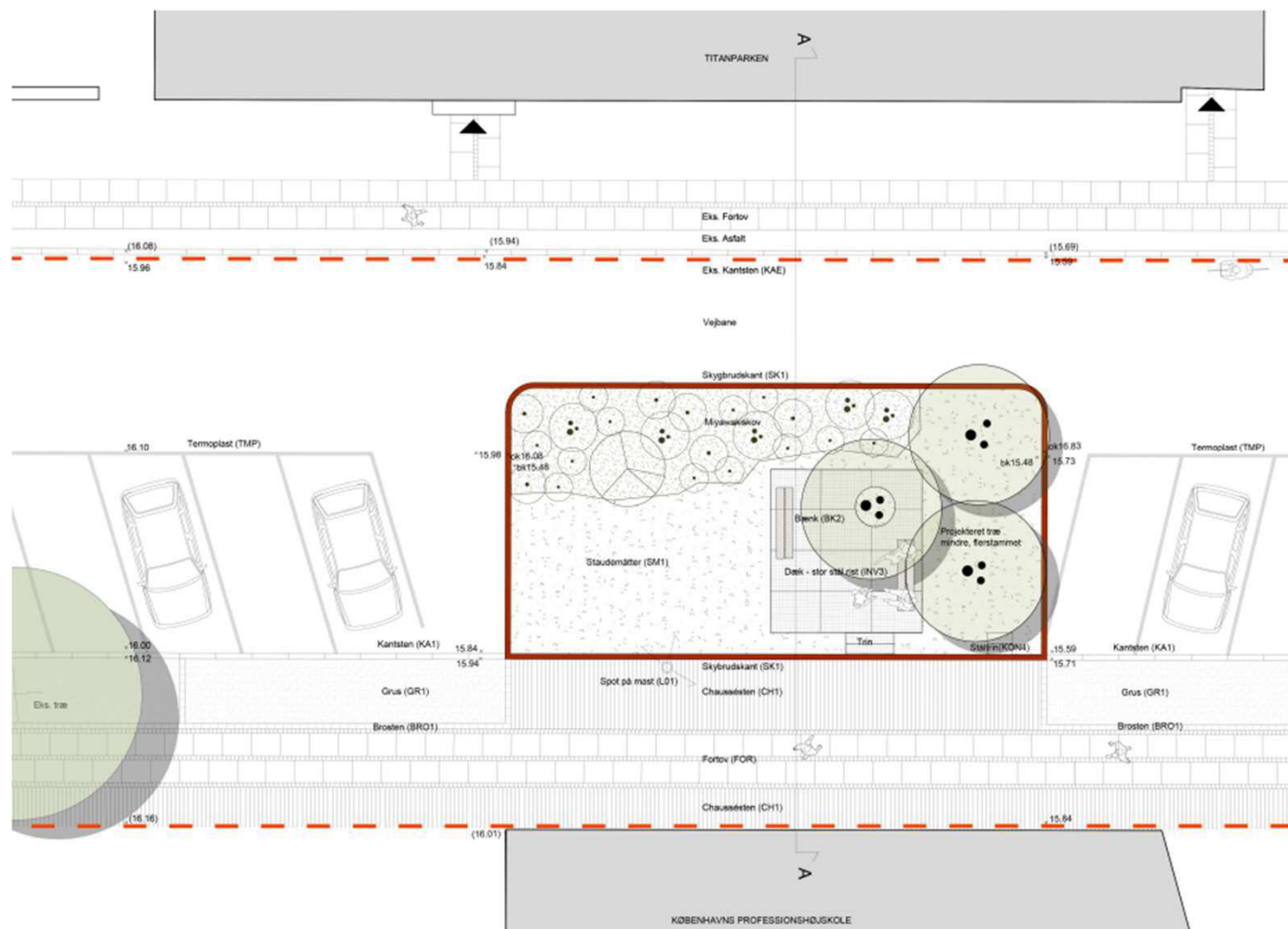
Planudsnit Sidegade med regnbed
