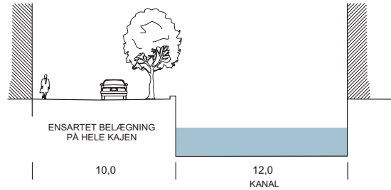
Snit D-D
