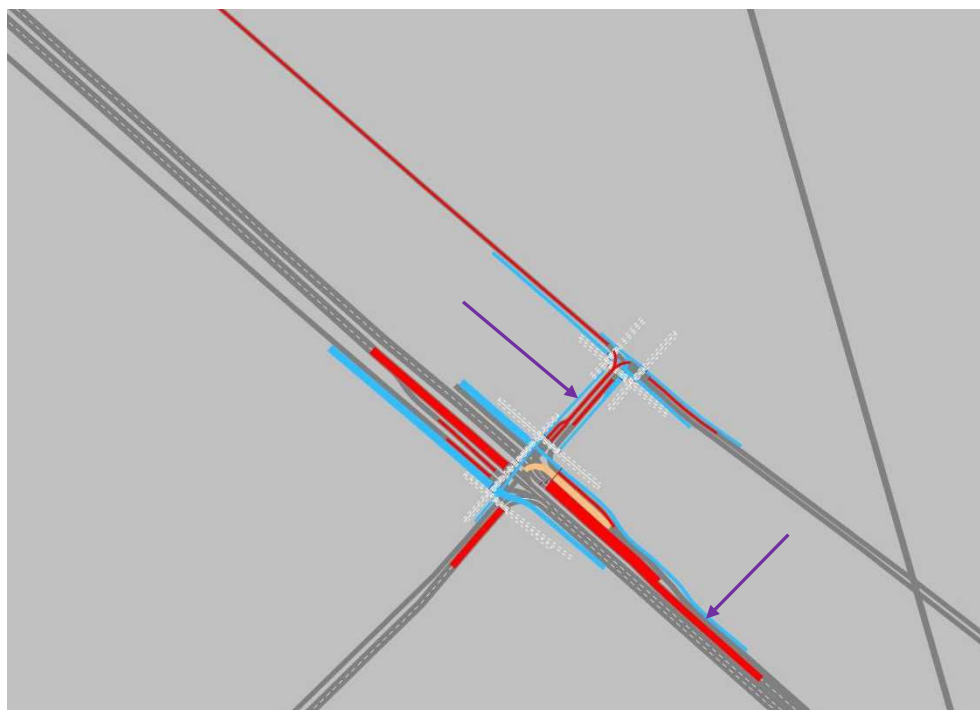
Figur 92 Figuren viser den maksimale kølængde (rød) i scenarie 1b ved krydset H. C. Andersens Boulevard / Rysensteensgade i morgenspidsperioden (kl. 7:00-9:00) [95% frakti- len].
