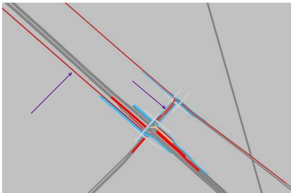
Figur 87 Figuren viser den maksimale kølængde (rød) i scenarie 1a ved krydset H. C. Andersens Boulevard / Rysensteensgade i morgenspidsperioden (kl. 7:00-9:00) [95% fraktile].
