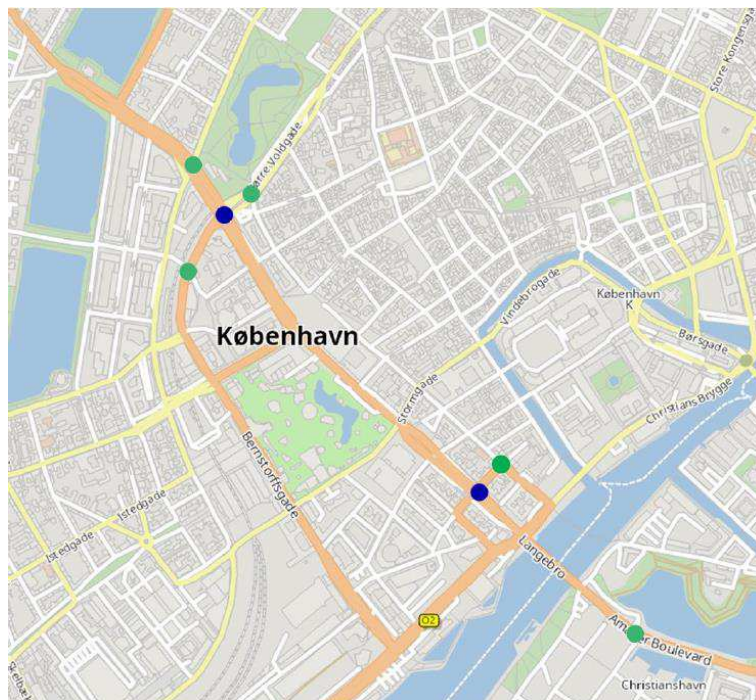
Figur 9 Figuren viser krydsene som er medtaget i simuleringsmodellen i VISSIM (blå – rampekryds, grøn – "dosseringsanlæg")
