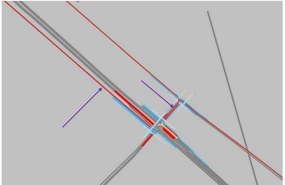
Figur 88 Figuren viser den maksimale kølængde (rød) i scenarie 1a ved krydset H. C. Andersens Boulevard / Rysensteensgade i eftermiddagsspisperioden (kl. 15:00-17:00) [95% fraktilen].
