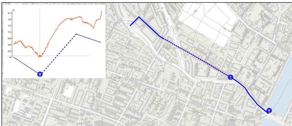
Figur 11 - Skitse af mulig linjeføring af søvandsledningen. Den stiplede delstrækning skal pumpes. Placeringen af de to pumper er markeret med blå cirkler.
