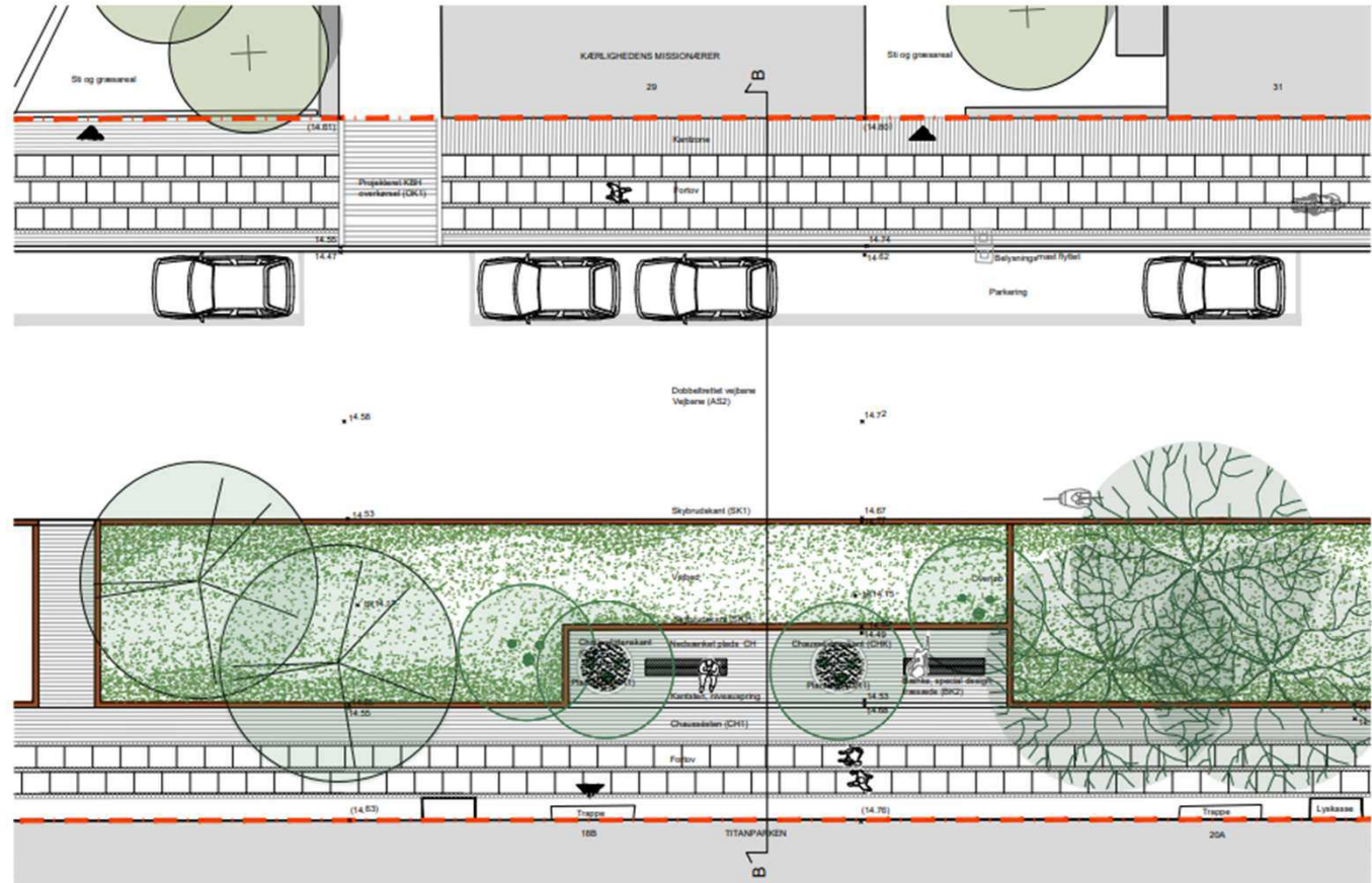
Planudsnit - Sigurdsgade med regnbed
