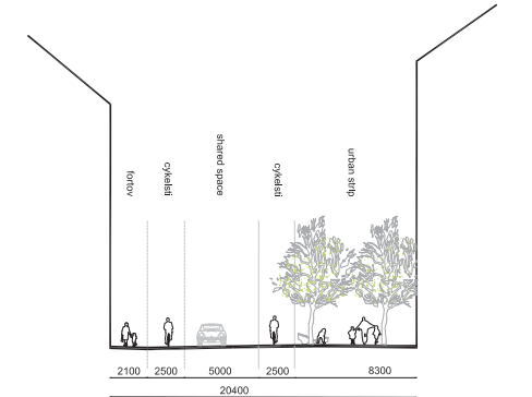
tværsnit ved Den Classenske Legatskole
