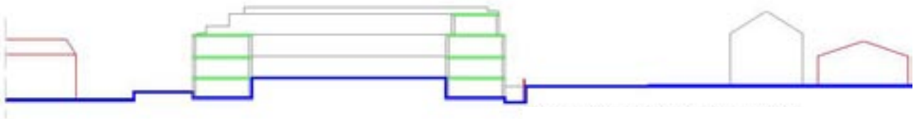
Principalsnit, eksisterende forhold
