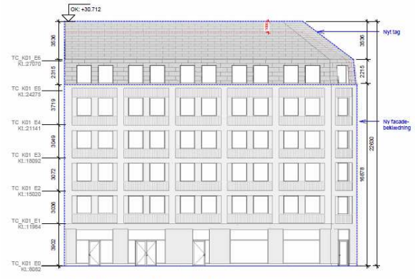
Vest - fremtidige forhold
