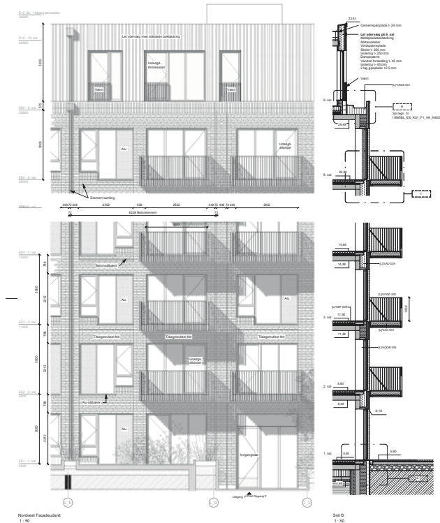
Facade udsnit
