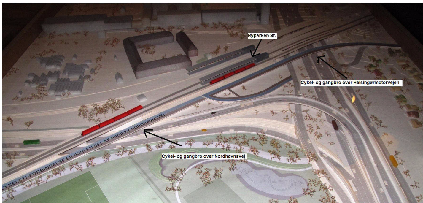
Model af broløsningen over Helsingørmotorvejen og Nordhavnsvej ved Ryparken St. Det blå og grå forløb illustrerer, hvordan Nørrebro-ruten fra højre føres først over Helsingørmotorvejen/Lyngbyvej og derefter over Nordhavnsvej. Ved Ryparken St. bygges desuden en rampe ned til stationen. 1
