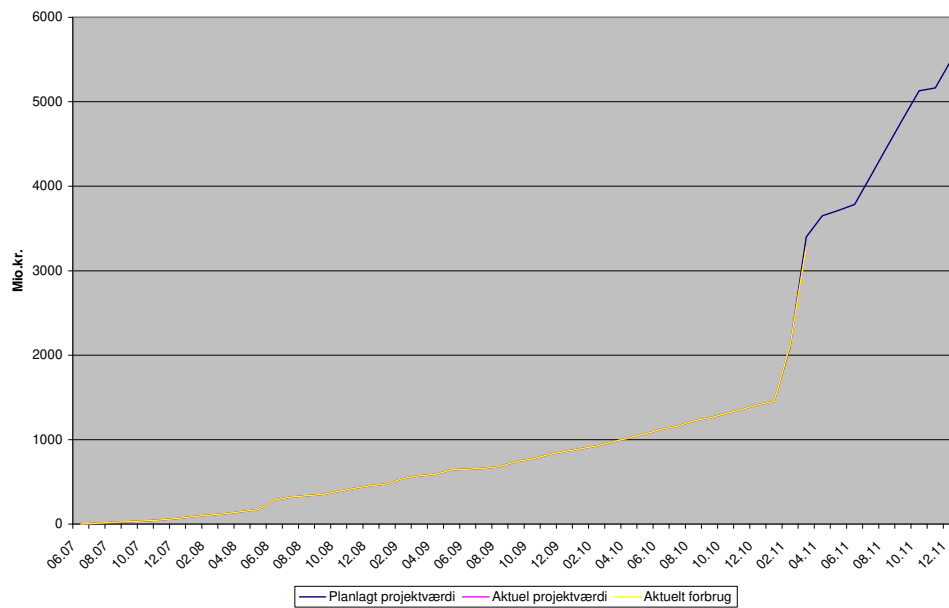
Cityringen S-kurver for 2007-2011. Status 31. marts 2011
