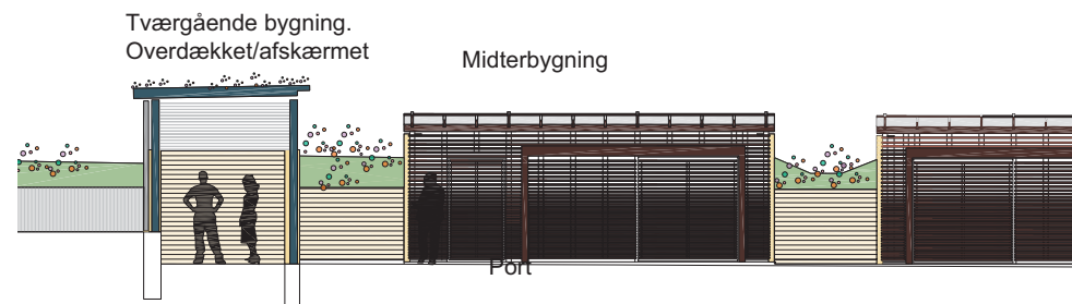
Opstalt/snit. Forslag 2..
