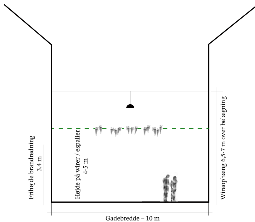
Snit gennem Frederiksberggade, 1:150
