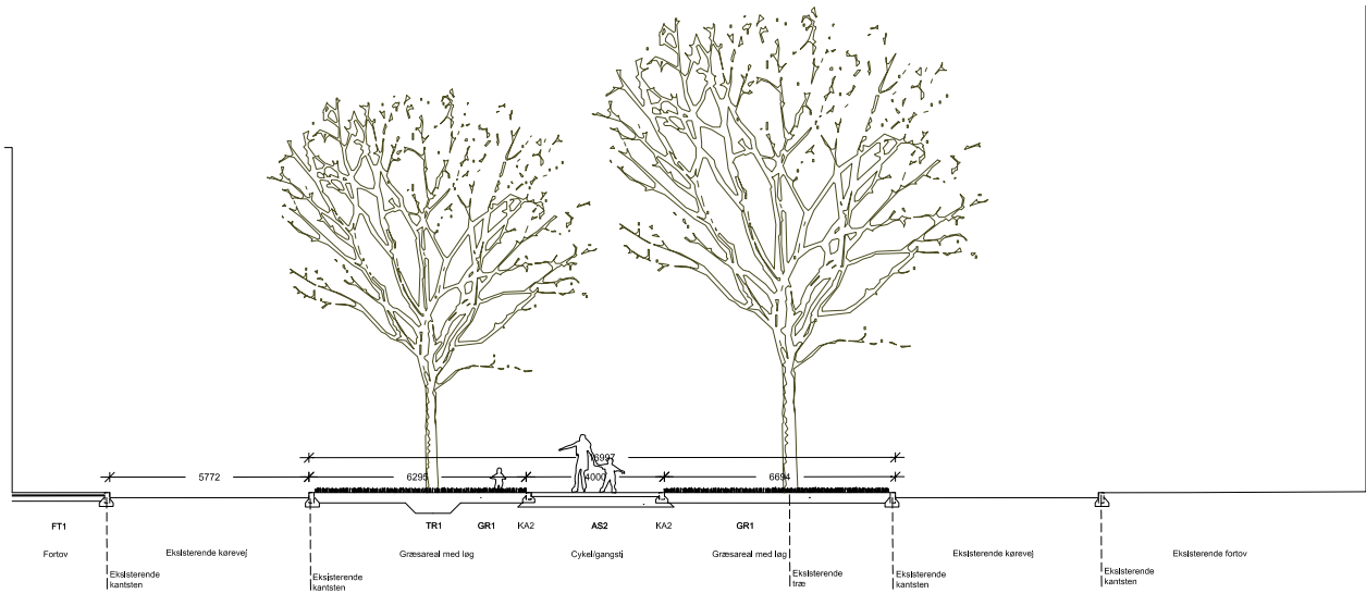
Snit gennem Lergravsvvej på den grønne del
