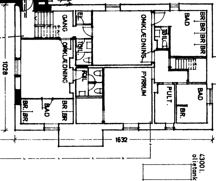
KÆLDERPLAN OMKLÆDNING OG BAD FOR V.B.C.
