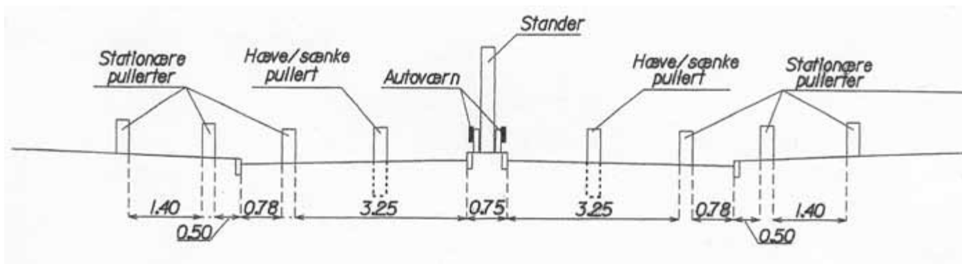
Tværsprofil, mål ca. 1: 100
