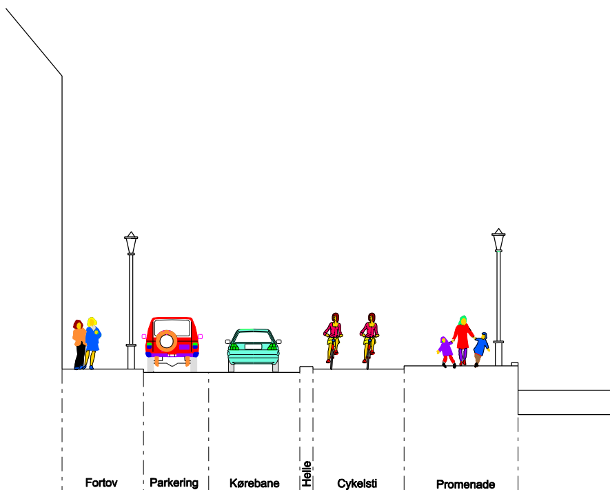
Tværprofil dobbeltrettet cykelsti
