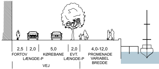
Snit C-C
