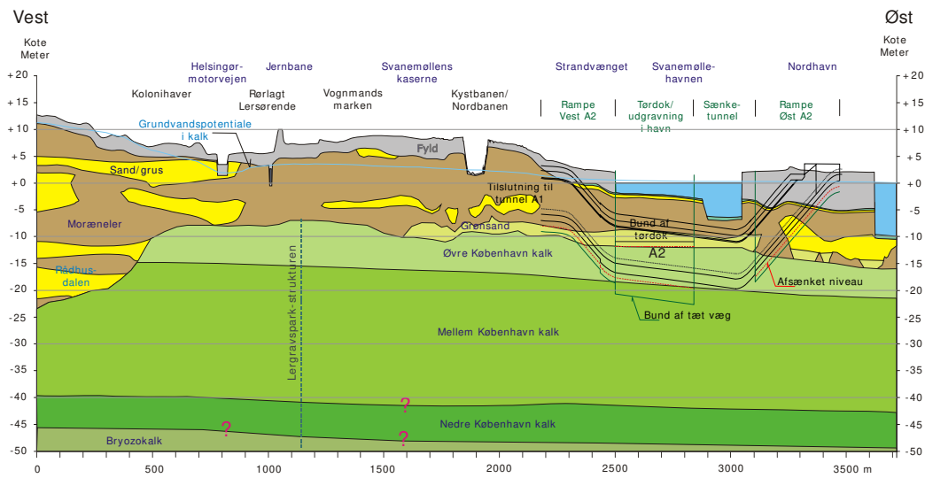
Figur 6.5 Geologisk længdeprofil for Vejforslag A2
