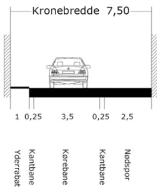
Figur 3.3 Tværprofil i til- og afkørsler ved Strandvænget i Vejforslag A2
