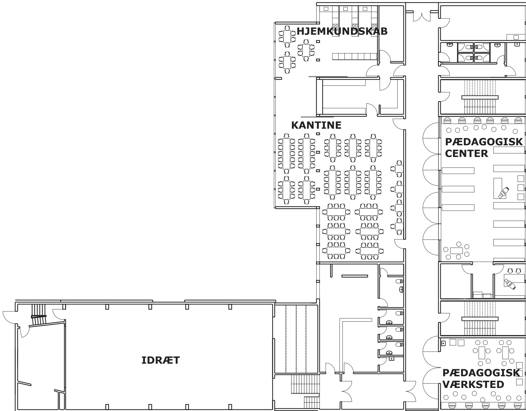
GASVÆRKSVEJENS SKOLE - BYGNING 2 - STUEETAGE - IDRÆT/PÆD. CENTER/KANTINE - KHR ARKITEKTER AS
