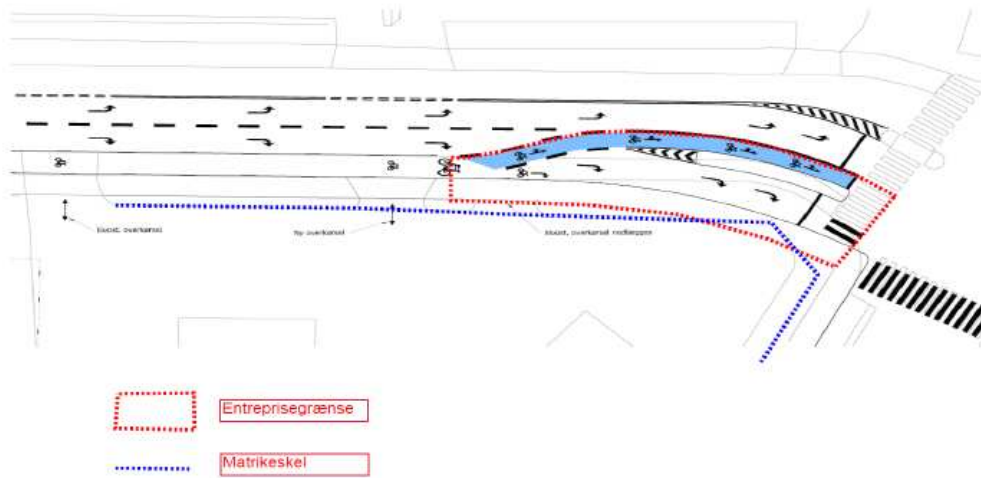
Figur 5-9 – Etablering af cykelbane i krydset Bådehavngade/Sjællandsbroen
