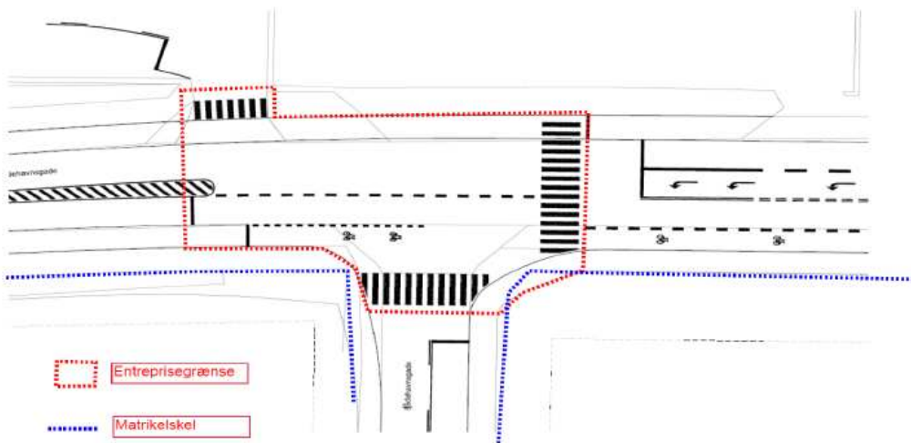
Figur 5-10 – Etablering af lyssignal Molestien/Bådehavngade.
