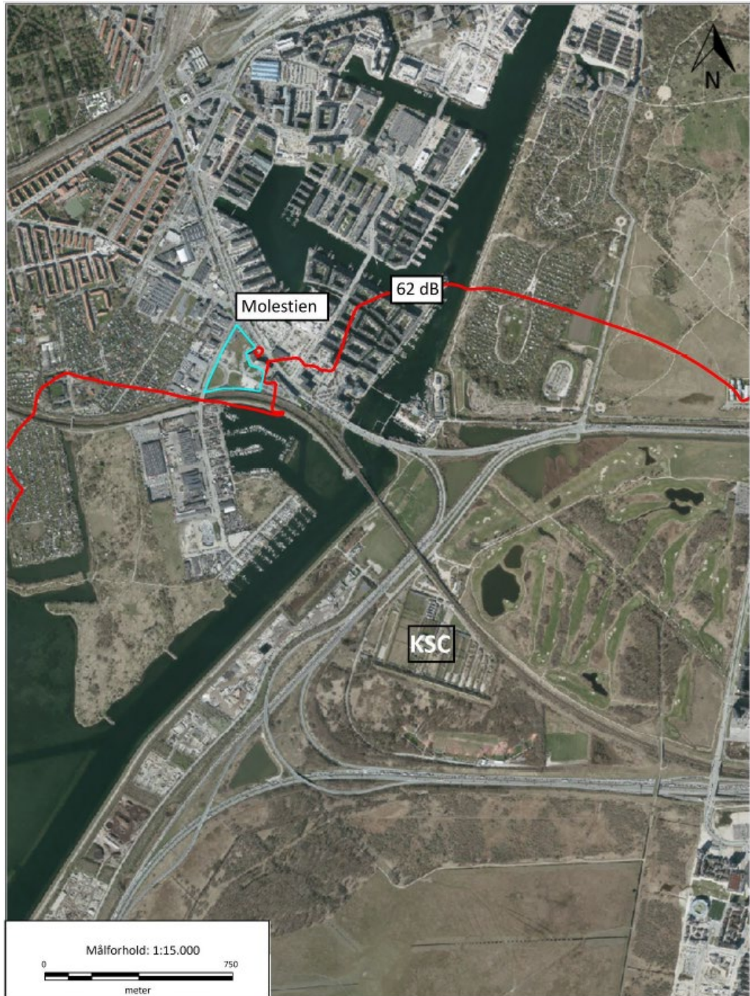
Figur 7-3: Støjubredelse fra Københavns Skyttecenter (KSC) hvis støjdem্পning udføres.
