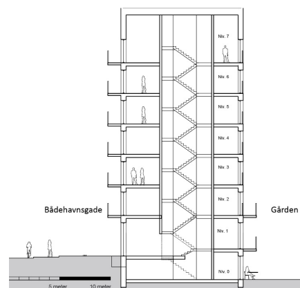
Snit, der viser håndtering af terrænspring i boligene langs Bådehavnsghade i overensstemmelse med lokalplanen. Illustration: DesignGroup Architects.
