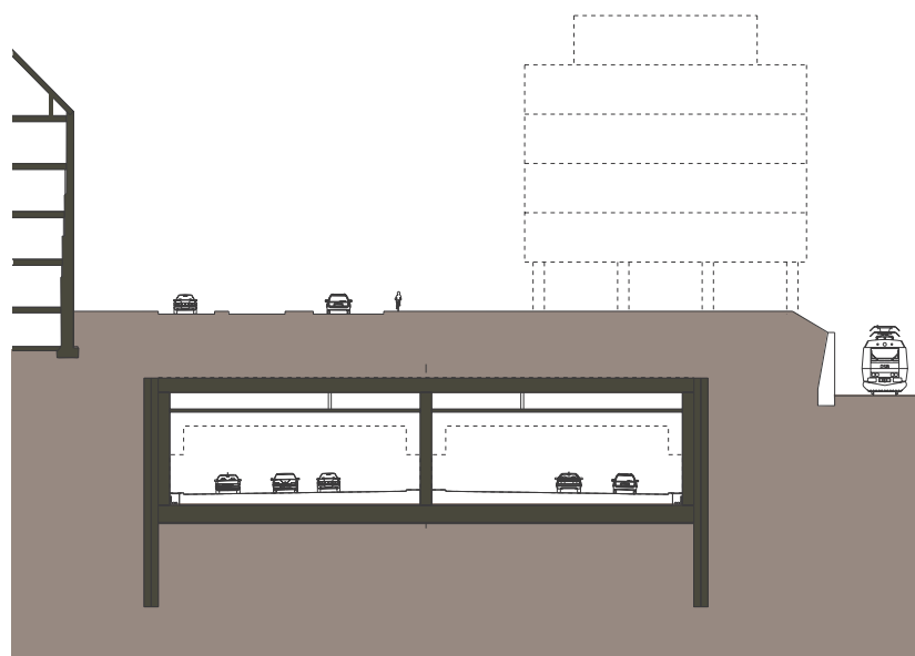
Figur 14. Tværsnit i Strandvænget ved Strandvejen. To spor plus nødspor og afkørsel til Strandvænget.
