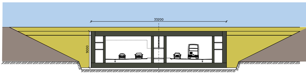
Figur 13. Tværsnit ved sænketunnel, 4 spor med almindelige nødspor (2,5 m.)
