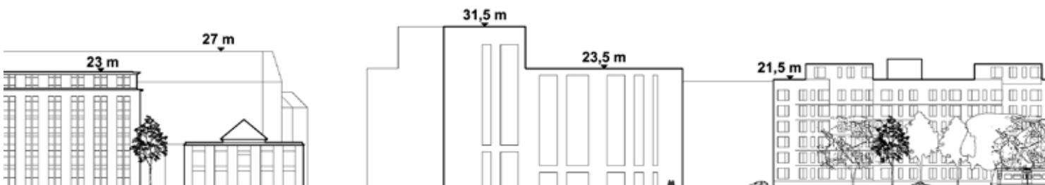
Opstalt set fra Jernbanens terræn med højdemål på den nye bygning og de eksisterende bygninger langs Kalkbrænderihavnsgade.
