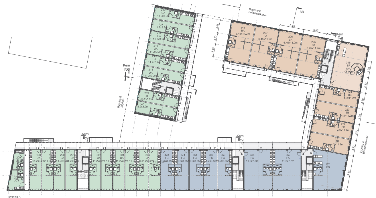
Etageplan med 4 boligtyper
