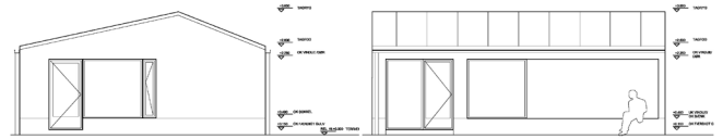
Facader fælleshus
