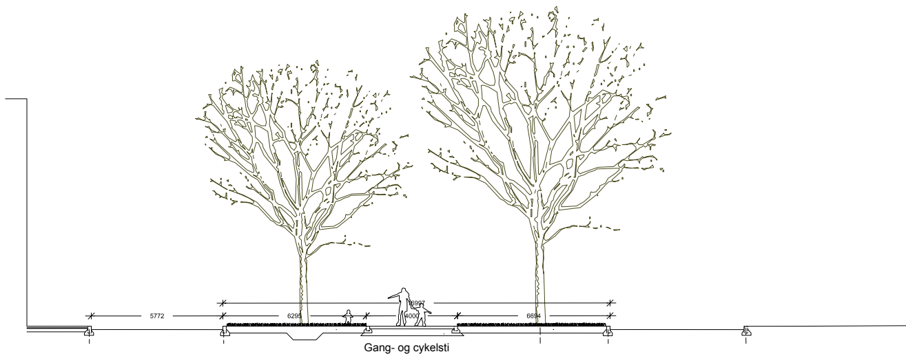
Lergravsvej. Snit i den grønne del med allétræer
