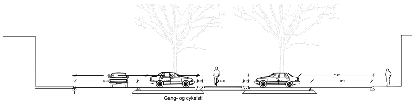
Lergravsvej. Snit i den grønne del med allétræer
