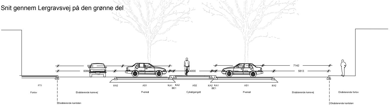
Snit gennem Lergravsvej ved parkeringspladserne
