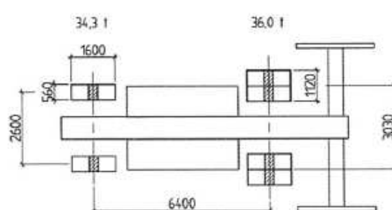
Aksellast, ubelastet
