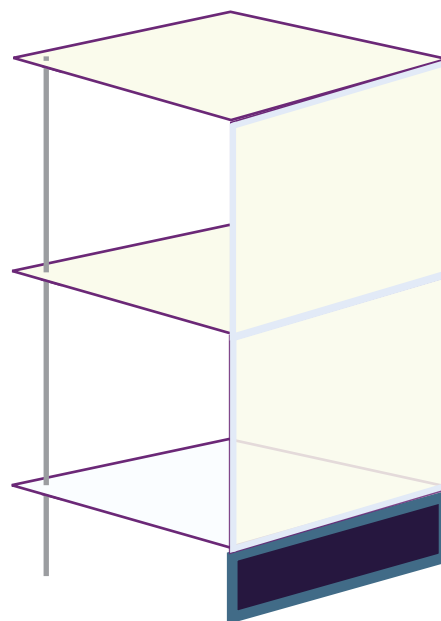
Tværsnit af detalje. Kasserne holdes på plads og sikres med 6 mm wire fastgjort i top og bund. Denne skjules af 35 x 35 mm alu-profil monteret udvendigt.
