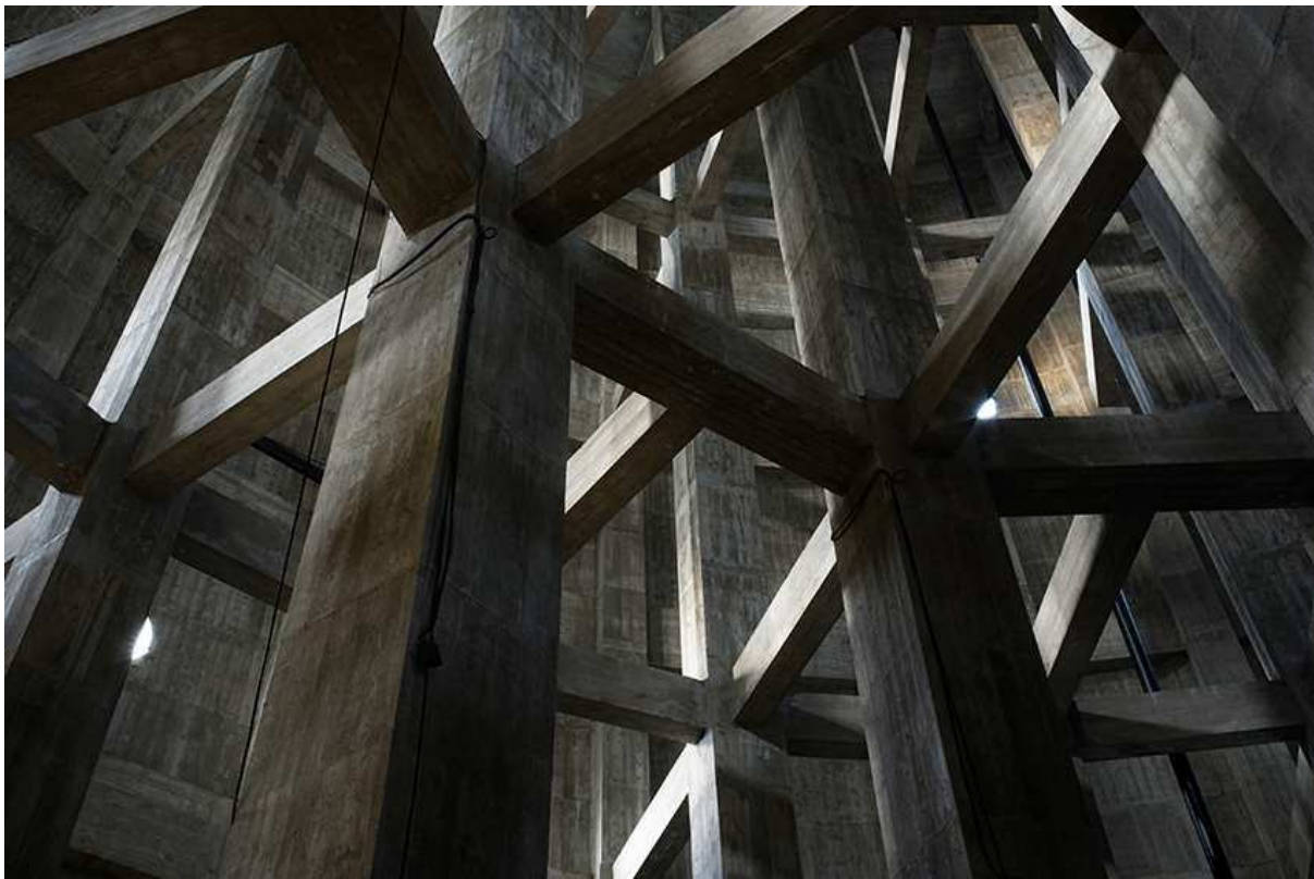
Interiør Brønshøj Vandtårn, 34m høje søjler
